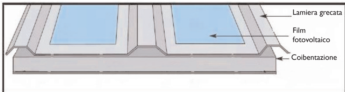
Figura 3. Modulo fotovoltaico non convenzionale consistente in film fotovoltaico su strato metallico sovrapposto a un pannello di coibentazione termica
